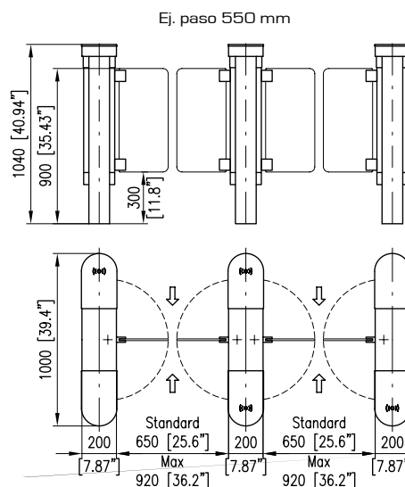
(Todas las dimensiones en mm y/o pulgadas)
