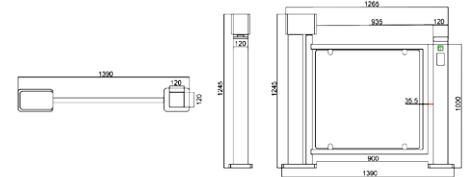
QRD-6003C Dimensions (mm)
